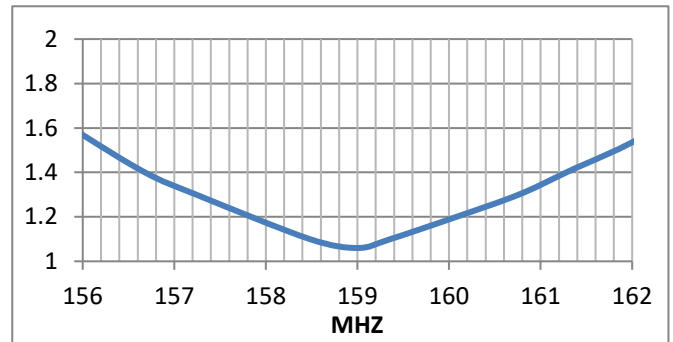
VSWR
