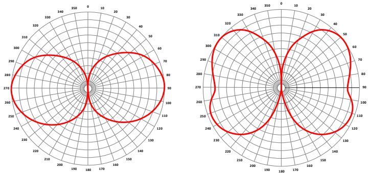
E-plane 860 MHz
