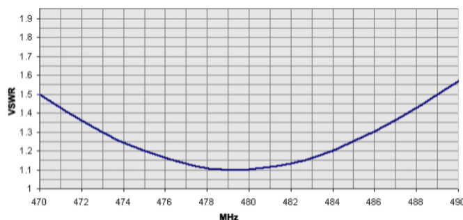
Typical VSWR Actual 02637X
